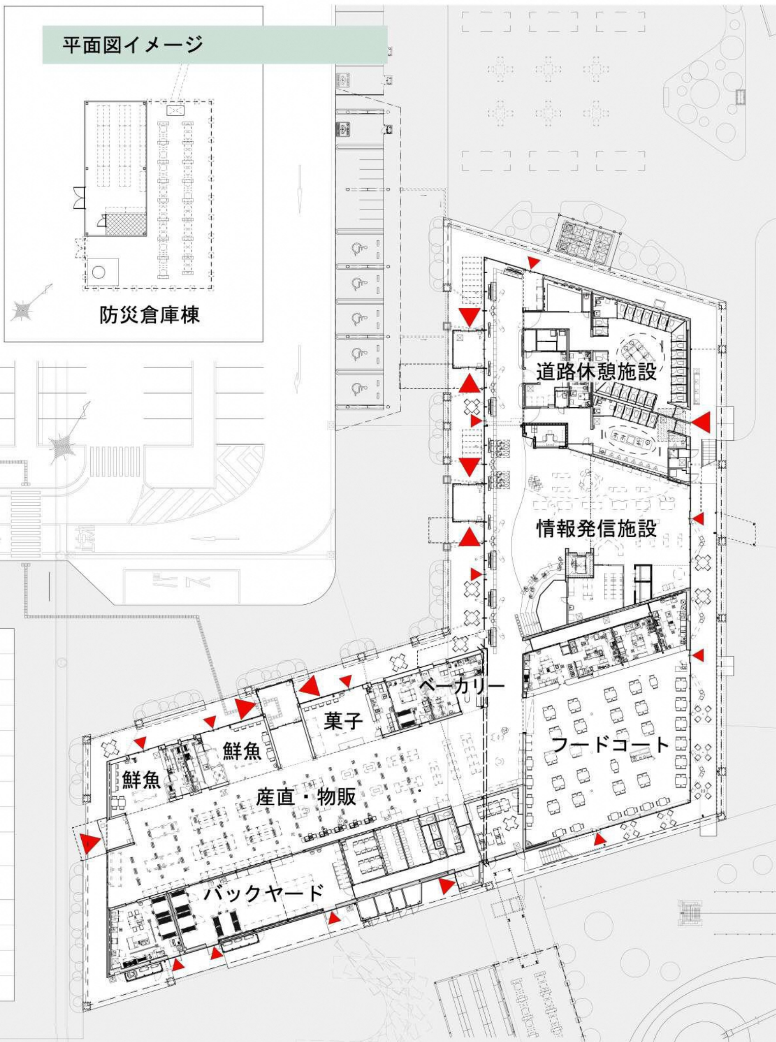
1 階平面図
